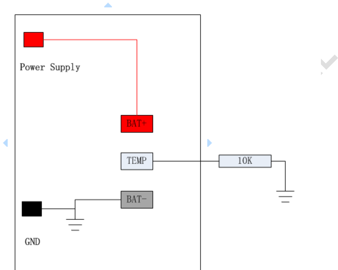
图 4.2 NTC 夹具接线方法
