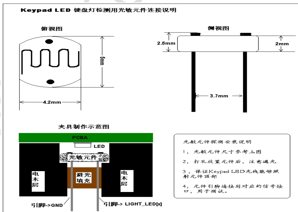
图 4.1 键盘灯检测光敏元件连接
